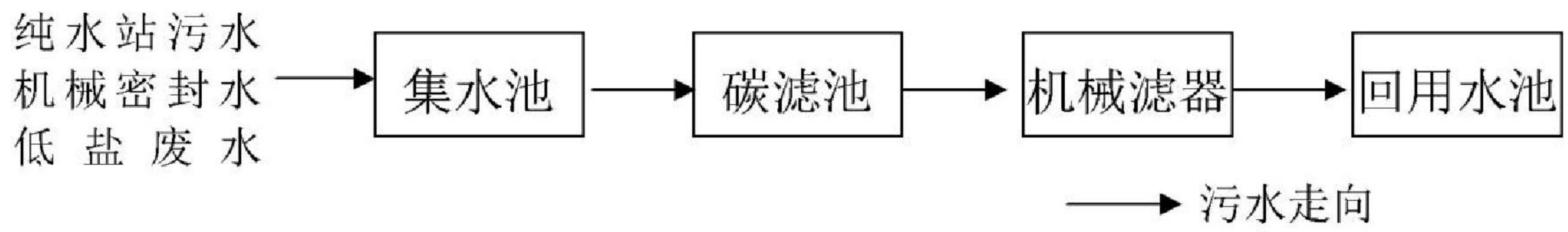
图 3-1 低盐废水处理工艺流程图
